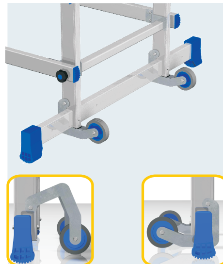
Base stabilizzatrice e ruote Stabilizer base and wheels
