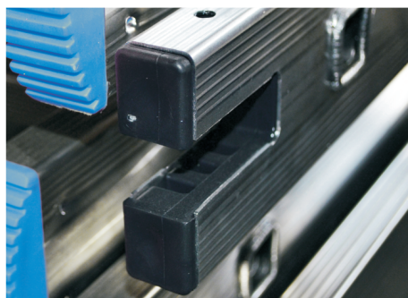
Agevolatore inserimento base stabilizzatrice Facilitator for insert stabilizer base
